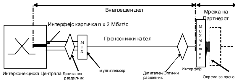
Слика 2. Внатрешен дел за интерфејс од 34 Mbit/s (E3) или 155 Mbit/s (CTM-1)
